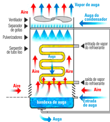
Fonte: Foto cedida por Baltimore Aircoil Iberica, S.A. Esquemas modificados da "Guía para la prevención de la legionelosis en instalaciones de riesgo". Comunidad de Madrid.
